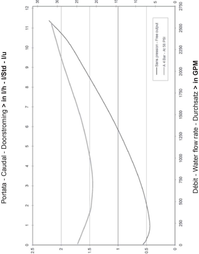
Perdite di carico - Perdidas de carga - Drukverlies > in Bar (kgf/cm²) © DOSATRON INTERNATIONAL / 219
